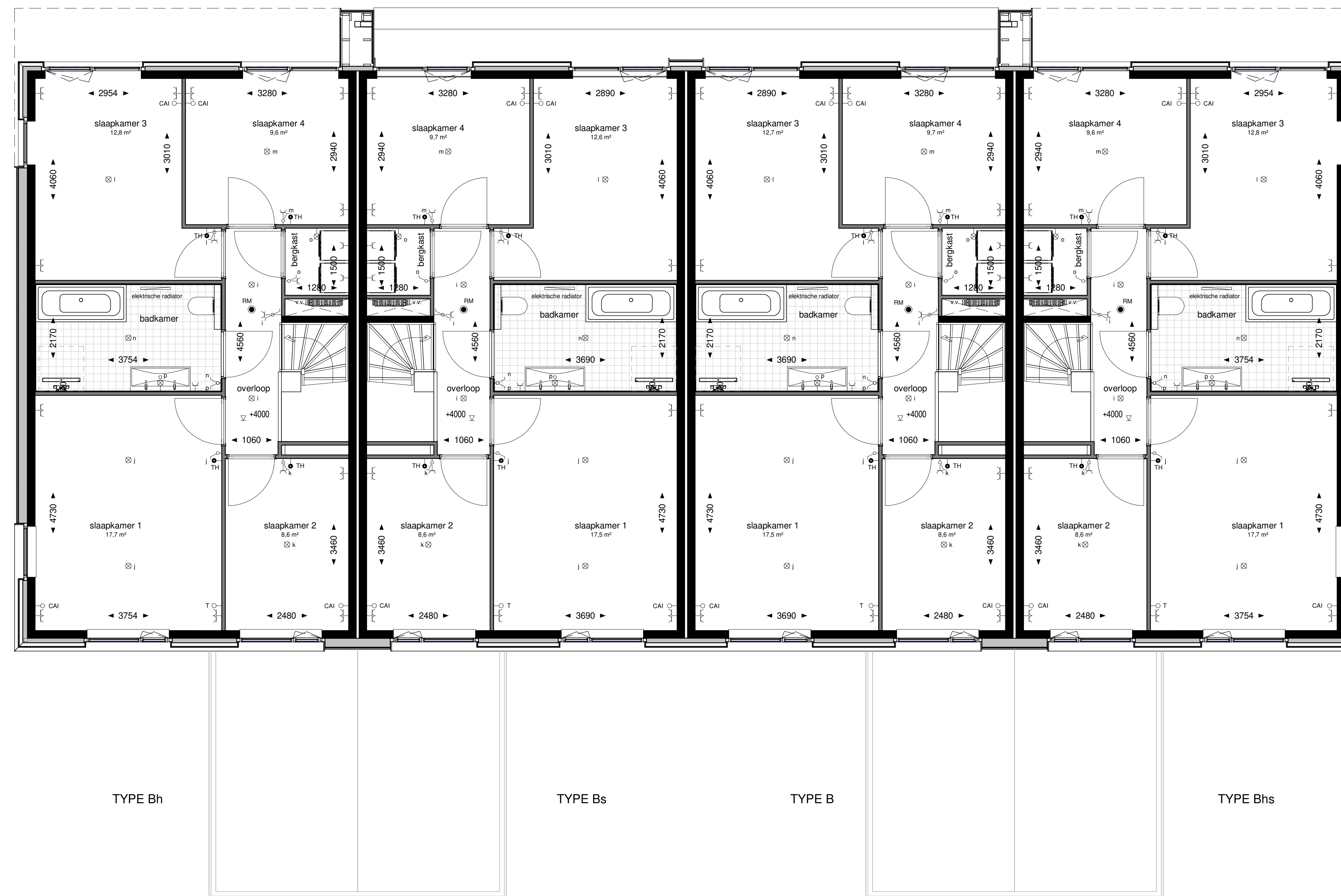
eerste verdieping 1 : 50
